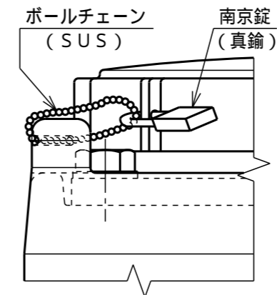
施錠仕様 (オプション)
