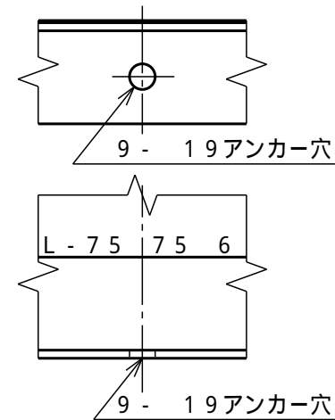
アンカ - 穴詳細
