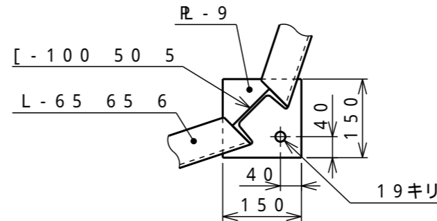
アンカー穴詳細
