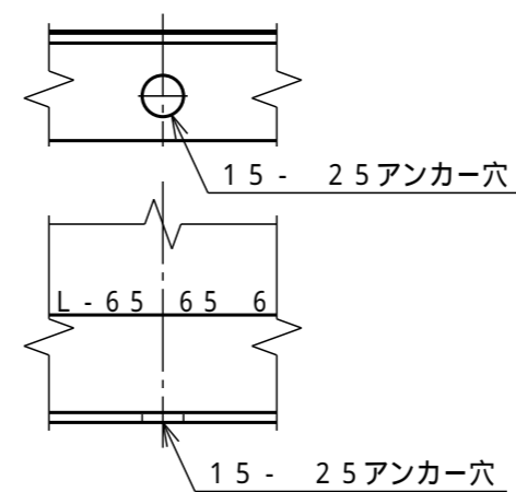
アンカー穴詳細
