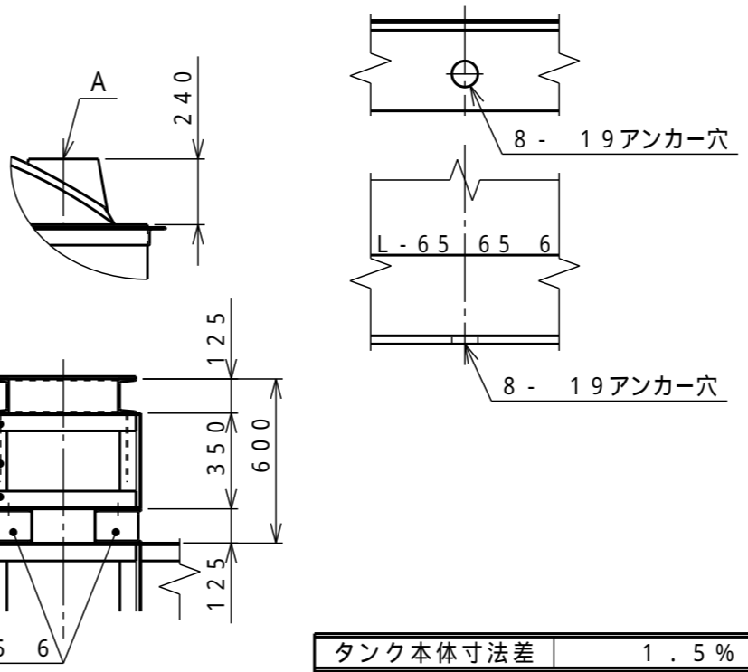
アンカー穴詳細
