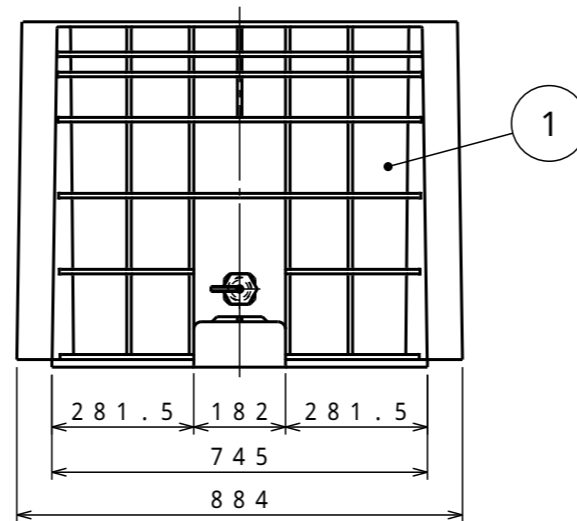
目盛部矢視
