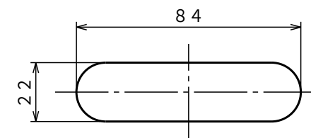
穴の寸法 (1:2) (8穴)
