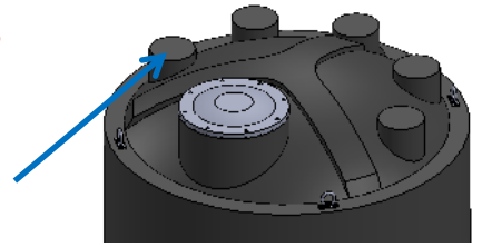
天板ノズル取付座 5ヶ所
